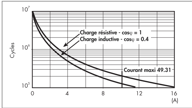
F 49 - Durée de vie électrique (AC) en fonction de la charge Types 49.31/61/81
