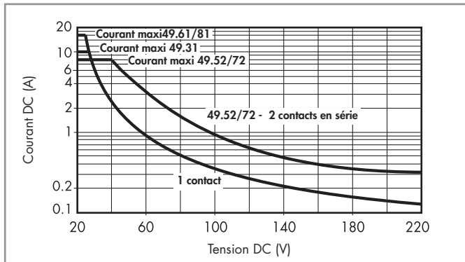
H 49 - Pouvoir de coupure maxi pour une charge en DC1 Types 49.31/52/61/72/81
