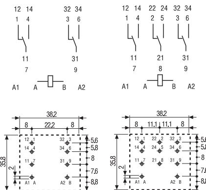
62.22 Vue coté cuivre
