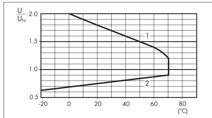
R 50 - Plage de fonctionnement bobine DC en fonction de la température ambiante, bobine standard (type 50.12)
