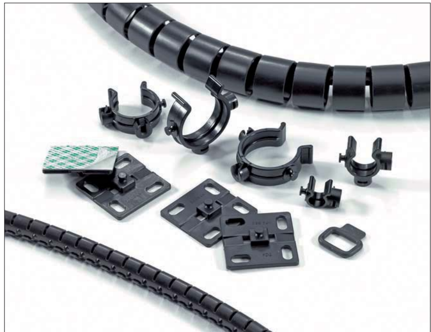
Le jeu d'accessoires clips et embases Helawrap pour maintenir, fixer et protéger des câbles multiples.
