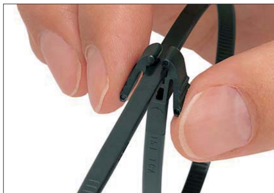
Les colliers REZ sont très faciles à réouvrir d'une seule main.
