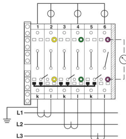
Circuit d'essai triphasé triangle (transformateur de mesure)
