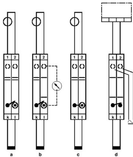
Circuit d'essai de transformateur d'intensité (simple)
