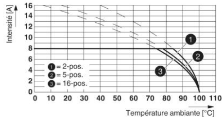
Type : MC 1,5/...-STF-3,81 avec DFK-MC 1,5/...-GF-3,81 (avec raccordement soudé)
