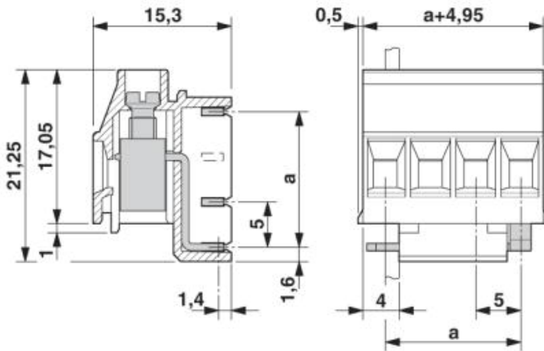
Dessin coté
