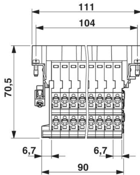
Dessin coté
