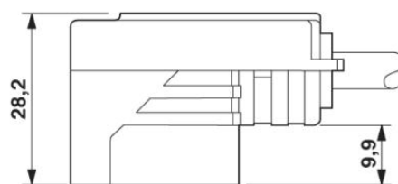
Connecteur pour électrovanne, type BI, vue latérale
