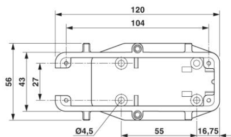
Dessin coté (vue de dessus)
