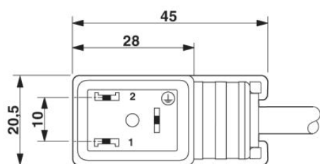
Connecteur pour électrovanne, type B
