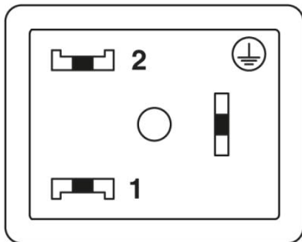
Schéma des pôles connecteur pour EV, type B
