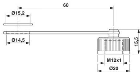
Dessin coté
