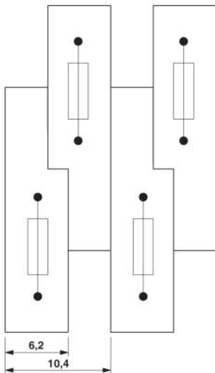
Blocs de jonction porte-fusibles interconnectés, module comprenant 5 blocs de jonction porte-fusibles
