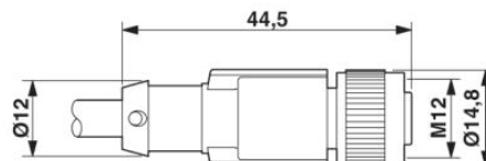
Connecteur femelle M12 x 1, droit, blindé
