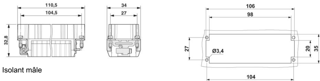
Découpe de montage
