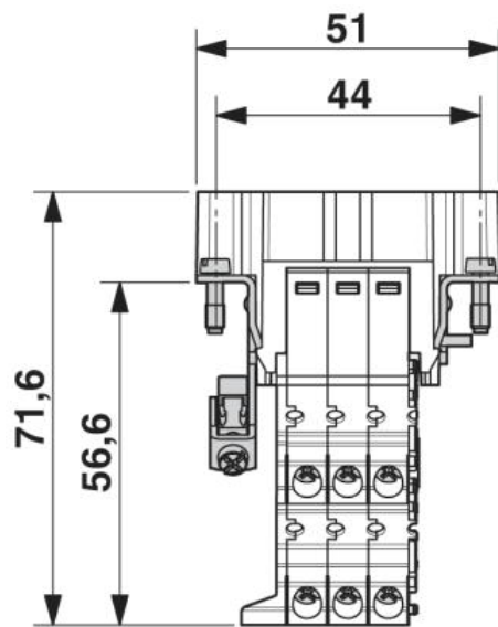
Côté raccordement
