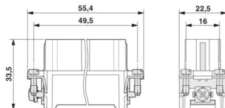
Isolant femelle
