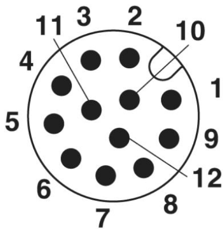
Schéma des pôles connecteur mâle M12, 12 pôles, côté mâle
