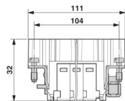
Isolant mâle
