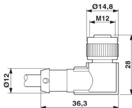
Connecteur femelle M12 x 1, coudé, avec LED
