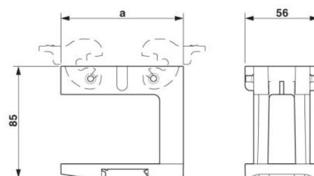
Dessin coté, a = 93,5 mm
