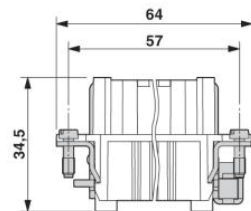
Isolant femelle
