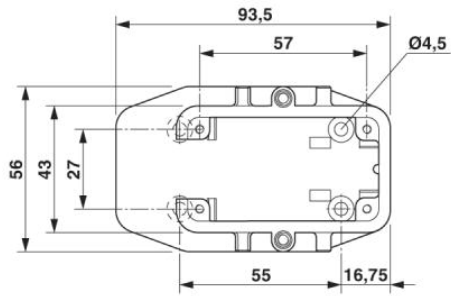
Dessin coté (vue de dessus)
