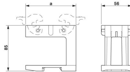
Dessin coté, a = 93,5 mm
