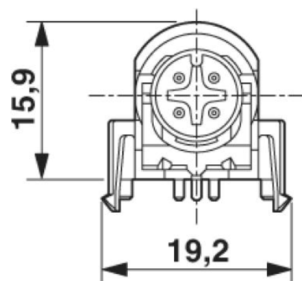
Connecteur encastrable M12, connecteur mâle, porte-contacts, vue de face
