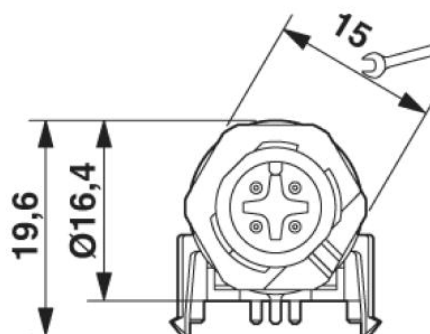
Connecteur encastrable M12, connecteur mâle, vue de face
