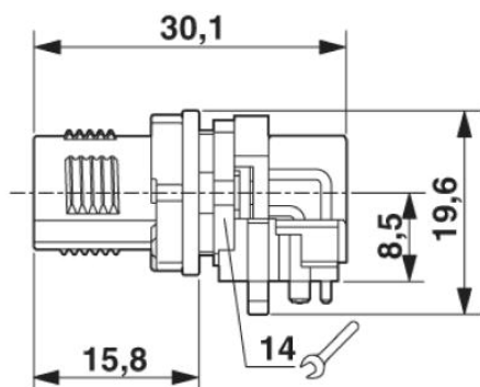
Connecteur encastrable M12, connecteur mâle, vue de côté
