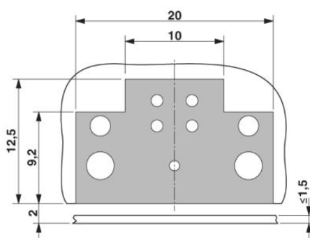
Surface verrouillée sur le C.I.
