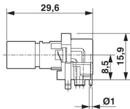
Connecteur encastrable M12, connecteur mâle, porte-contacts, vue de côté
