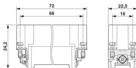
Isolant mâle
