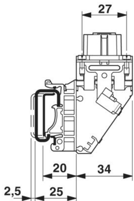
Dessin coté, vue de côté
