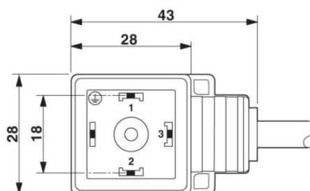
Connecteur pour électrovannes, type AD Connecteur pour électrovanne, type AD, vue latérale
