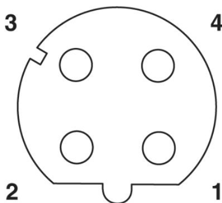
Dessin schématique
