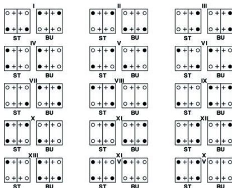
Débrayage pour capots avec deux isolants
