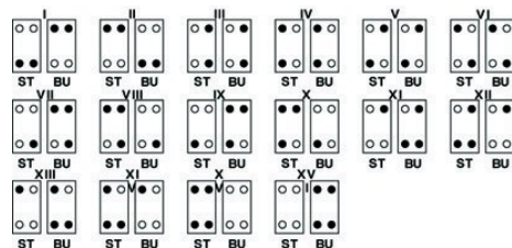
Débrayage pour capots avec un isolant
