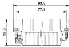
Isolant mâle
