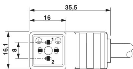
Connecteur pour électrovanne, type C
