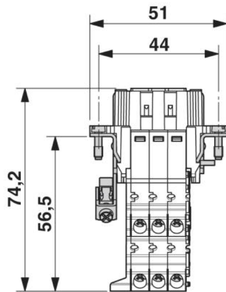
Côté raccordement
