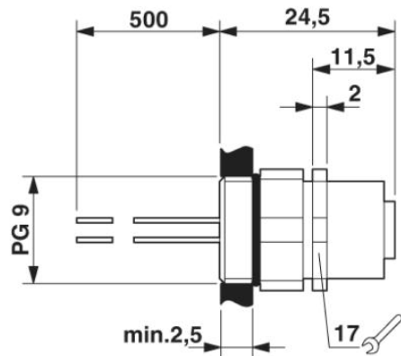
Connecteur mâle encastrable M12, positionnable
