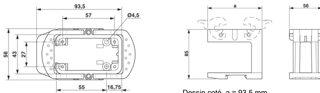
Dessin coté (vue de dessus)
