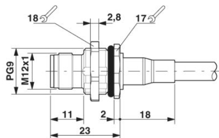
Traversée de paroi M12
