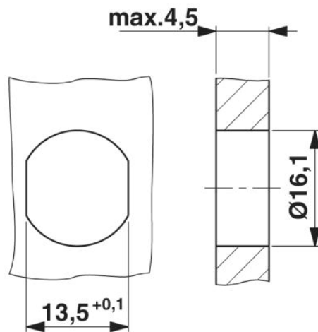
Découpe du boîtier pour filet de fixation Pg9, paroi de montage avec perçage traversant (alternativement avec surface de protection anti-torsion)
