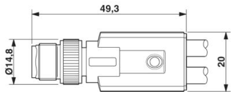
Connecteur mâle M12x1, répartiteur en Y
