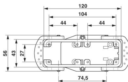
Dessin coté, a = 120 mm
