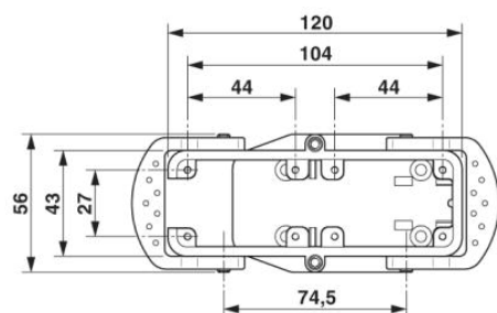
Dessin coté (vue de dessus)
