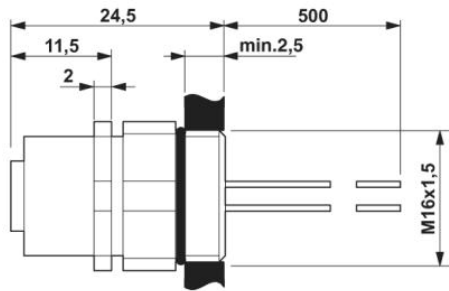
Connecteur femelle encastrable M12, positionnable
