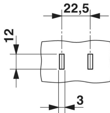
Gabarit de poinçonnage
