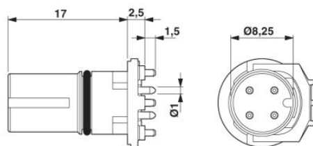
Porte-contacts femelle M12
