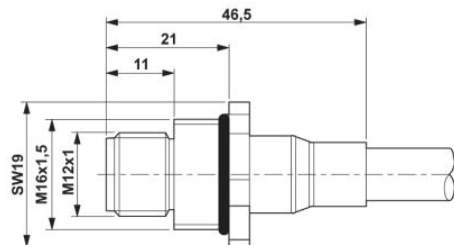
Connecteur mâle encastrable M12
