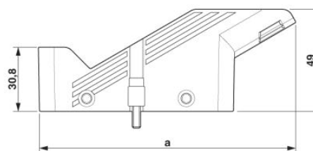
Dessin coté, a = 123,7
