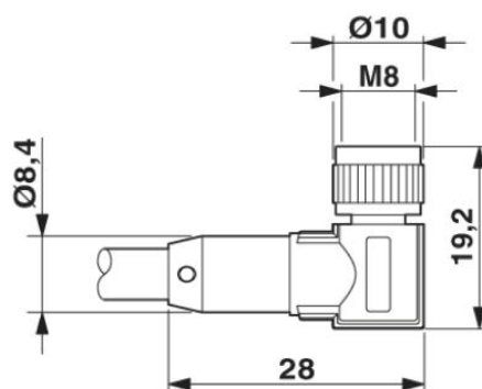
Connecteur femelle M8 x 1, coudé, avec LED
