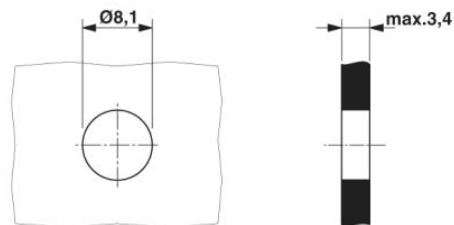
Découpe du boîtier pour connecteurs encastrables M8, connecteur mâle, 1 pièce
