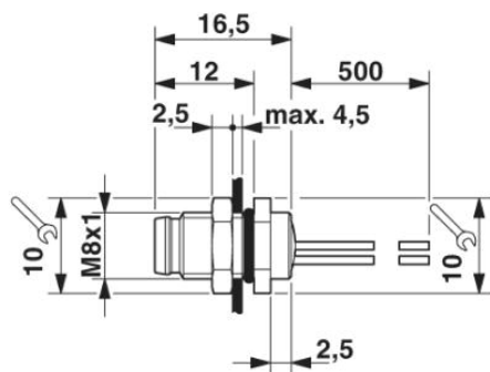
Connecteur mâle encastrable M8
