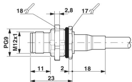
Traversée de paroi M12
