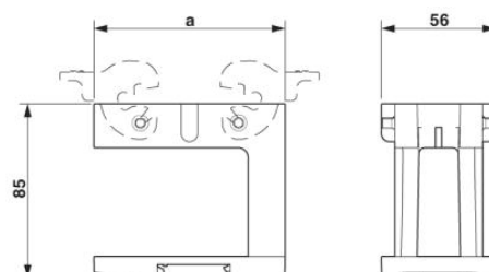
Dessin coté, a = 120 mm
