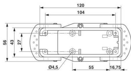
Dessin coté (vue de dessus)
