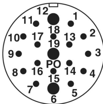
Raccordement enfichable M23 mâle, 19 pôles
