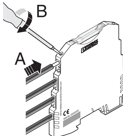
Fig. 4 Raccordement vissé
