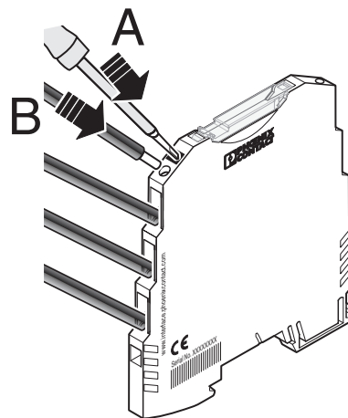
Fig. 5 Raccordement à ressort
