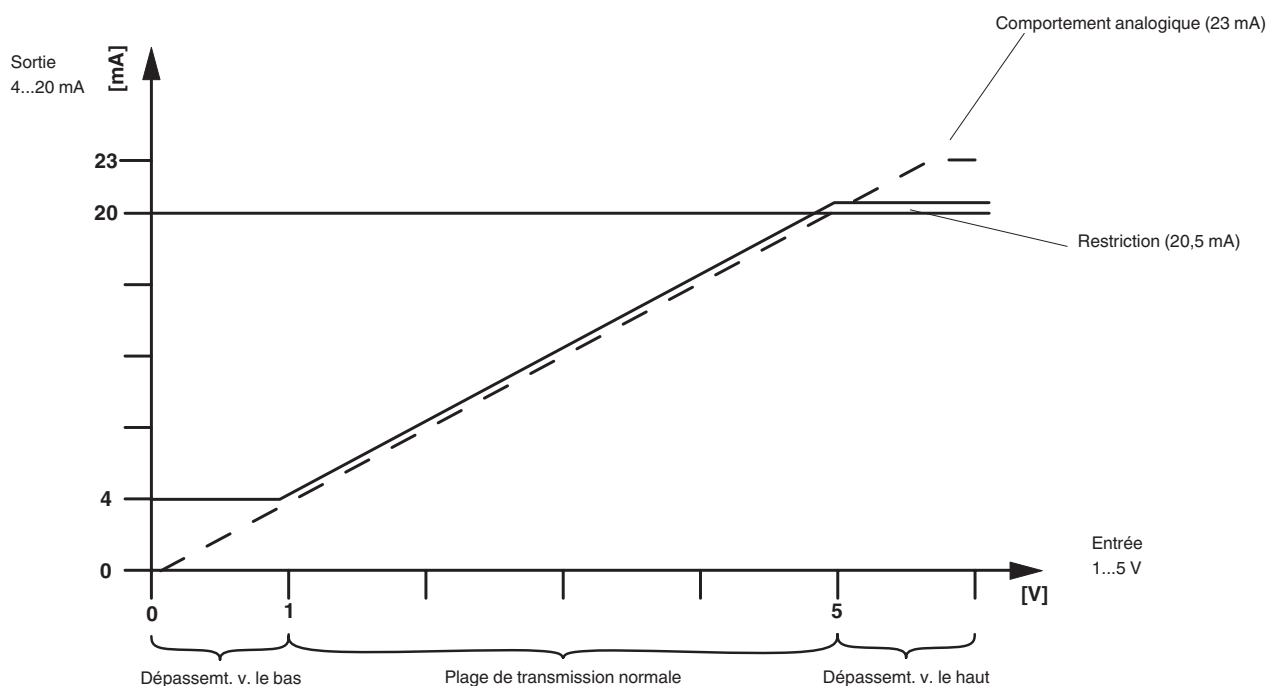
Fig. 6 Comportement des sorties analogiques
